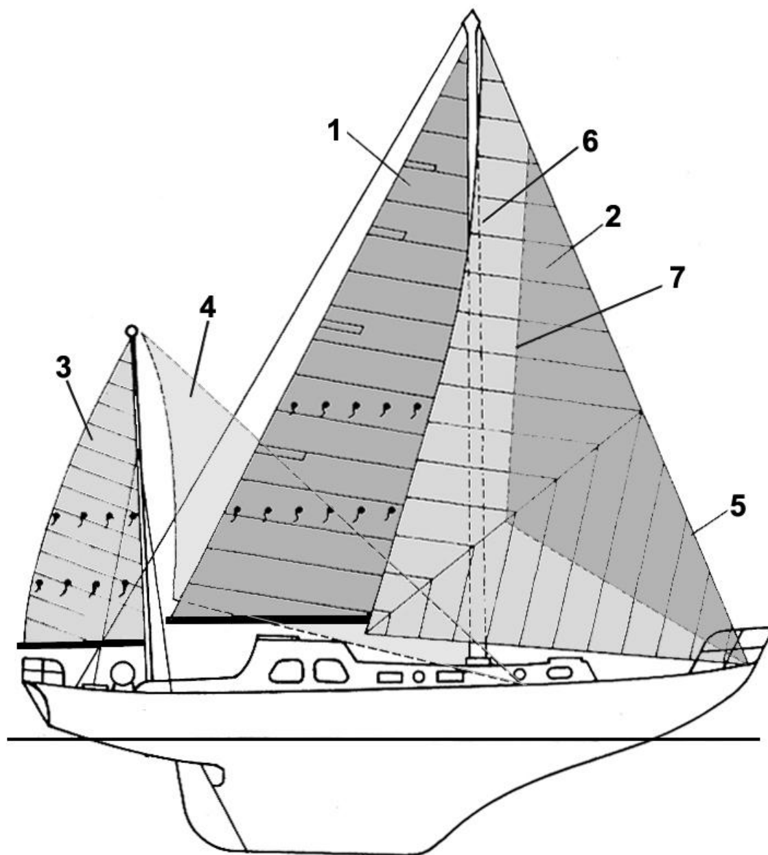
Ożagłowanie marszowe: 1 – grot, 2 – genua, 3 – bezan, 4 – apsel, 5 – forsztagi (dwa), 6 – fok, 7 – kliwer
